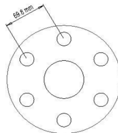
6 Stud
